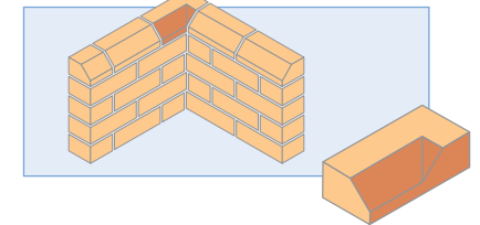
PL.3.1/PL.3.2 Plinth Stretcher
