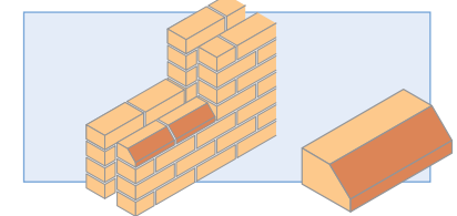
AN.5.1/AN.5.2 Single Cant
