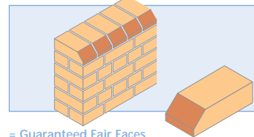
PL.2.1/PL.2.2 Plinth Header
