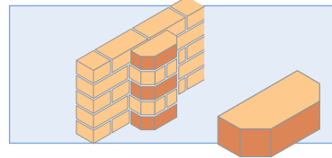
AN.2.2 45° External Angle
