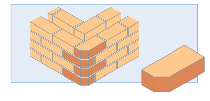
AN.5.1/AN.5.2 Single Cant
